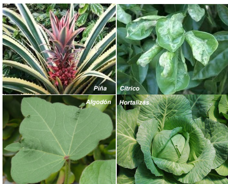
Figura 21. Tipos de hojas y la ET Fuente: www.google.com
