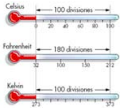
Figura 4. Escalas térmicas utilizadas Fuente: http://blnlaus.blogspot.com/
