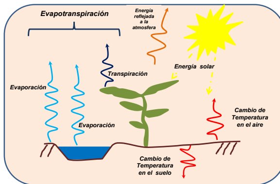
Figura 16. Componentes de la evapotranspiración Fuente: Watplan.com
