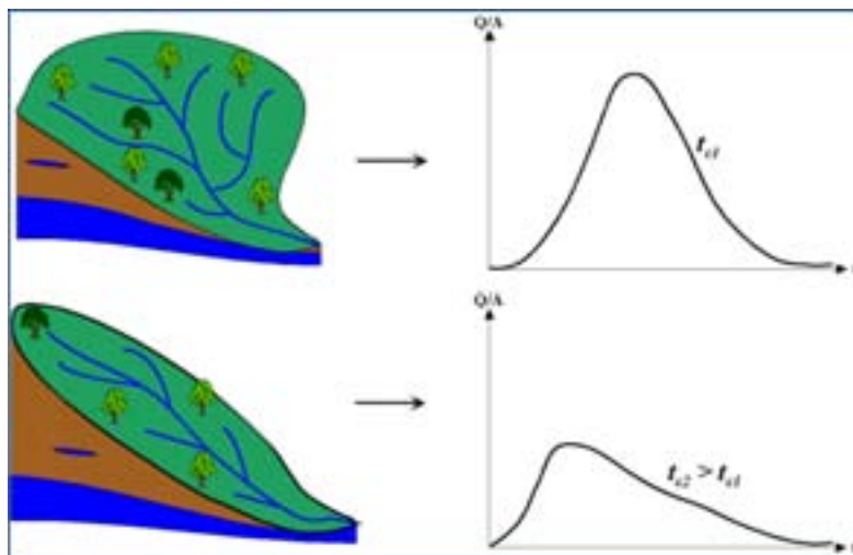
Figura 6. Tipos de hidrograma en función a la cuenca
