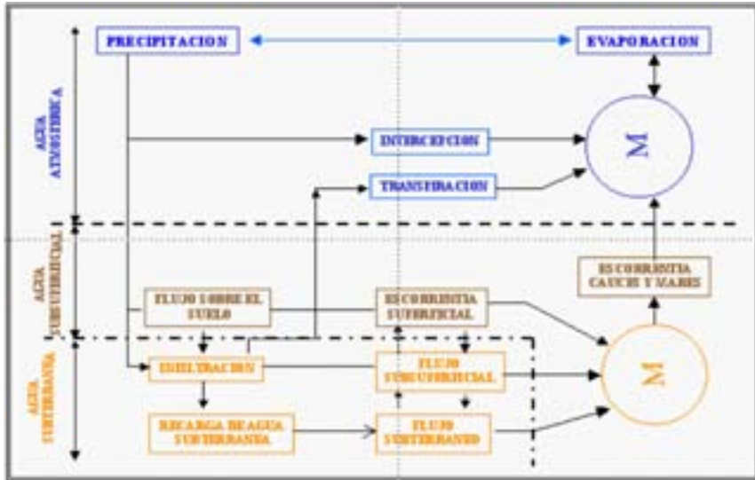
Figura 2. Representación del sistema hidrológico
