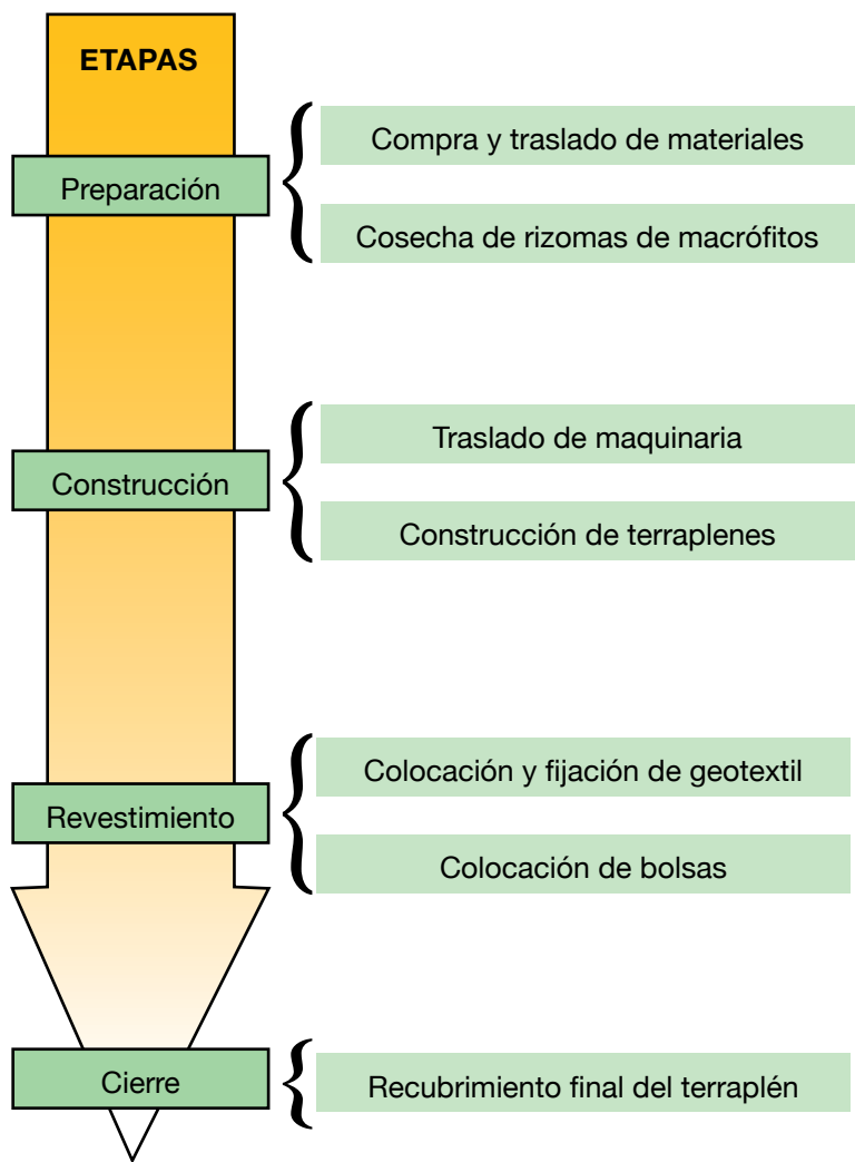
Figura 18.- Etapas y actividades para la ejecución de las obras.
