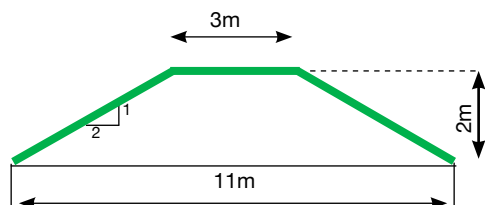
Figura 16.- Esquema de terraplén o azud nivelador.
