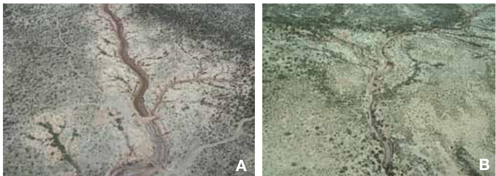
Figura 26.- Fotografía aérea de las obras de restauración: A) La Pasarela y B) La Puertita.
