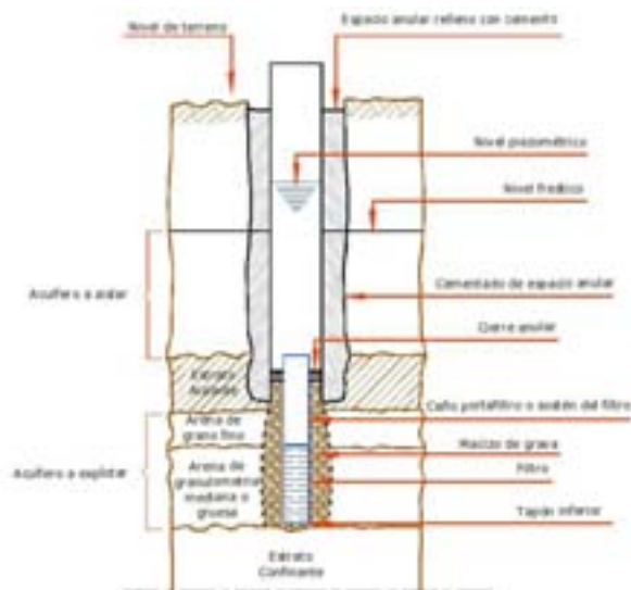
Figura 26. Perfil de un pozo artesiano Fuente: Bellino, 2012
