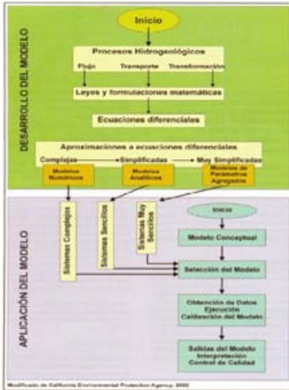
Figura 22. Esquema de Modelamiento de acuíferos.
